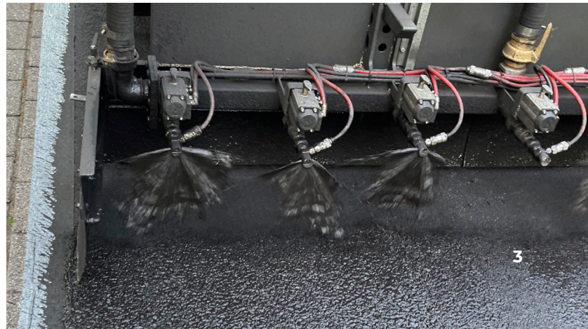
1 Onyxauftrag | 2 fertige Oberfläche | 3 Düsen-spritzvorrichtung
